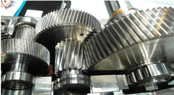
Ein schrägverzahntes Stirnradgetriebe, ein Kunstgenuss für den Ingenieur...
